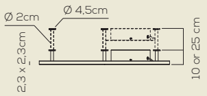
altezze disponibili available heights
